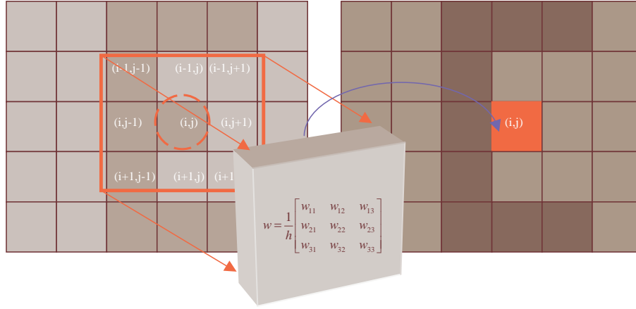
Figura 3.1: Filtrado espacial por una mascara de 3 x 3.
